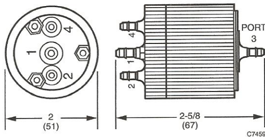
Fig. 1. RP971A Dimensions,
